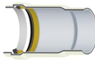
TOP-CONNECT Muffensystem
